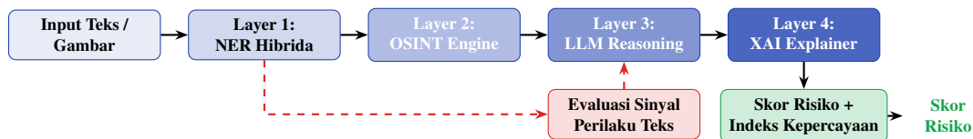
Gambar 5.1 Arsitektur Pipeline Analisis Verifin
